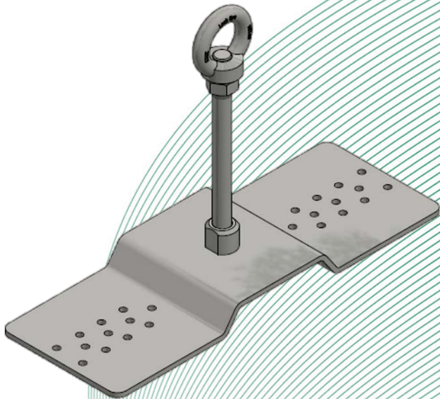
Figure 1 : Dispositif d'ancrage, type : ABS-Lock® X-SW-6
