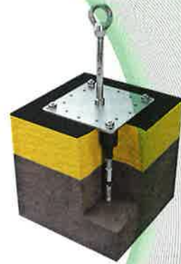
Figure 14 : Dispositif d'ancrage, type : ABS-Lock® X-Therm
