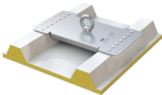
Figure 17 : Dispositif d'ancrage, type : ABS-Lock® X-Rivet
