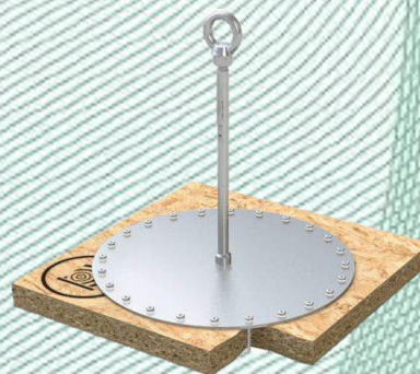
Figure 14 : Dispositif d'ancrage, type : ABS-Lock® X-H-24
