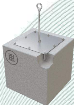
Figure 13 : Dispositif d'ancrage, type : ABS-Lock® X-Y
