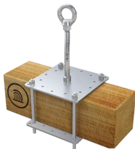
Figure 11 : Dispositif d'ancrage, type : ABS-Lock® X-Klemm
