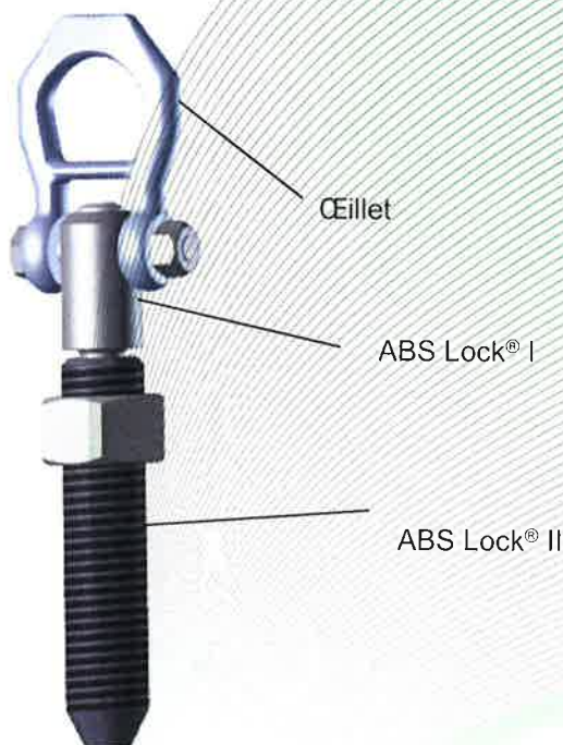
Fig. 1 : Dispositif d'ancrage avec manchon fileté
